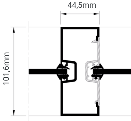
Vertical típico
