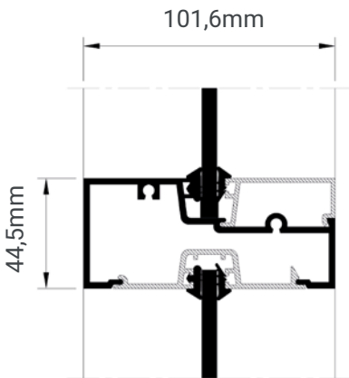
Horizontal típico
