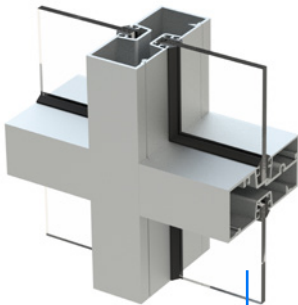
Corte isométrico
